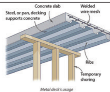
ỨNG DỤNG CỦA TẤM SÀN KIM LOẠI METAL DECK'S USAGE
